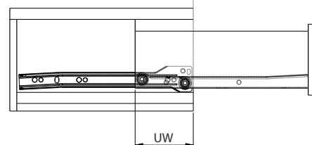
KRAWĘDŹ SZAFKI / CABINET EDGE
