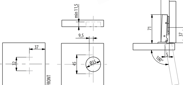
ZP03 - zawias do drzwi wpuszczanych / inset door hinge
